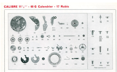
Calibre 11 1/2''' - 60 G Calendrier - 17 rubis [éclaté des fournitures du Parrenin HP 60 G], 1973. IVR43_20162500632NUC4A
