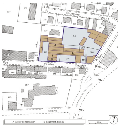
Plan-masse et de situation. Extrait du plan cadastral, 2001, section BC, 1:1000. Dess. André Céréza IVR43_20039000070NUDA
