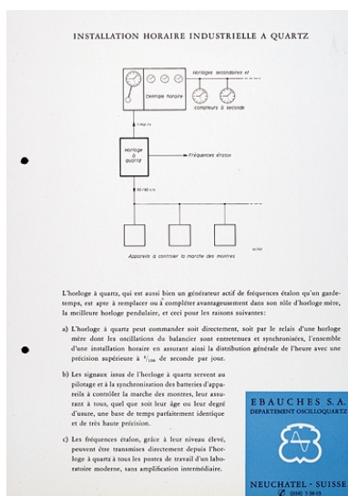
[Exemple d'appareil du département Oscilloquartz, Ebauches SA :] Installation horaire industrielle à quartz, vers 1955.
