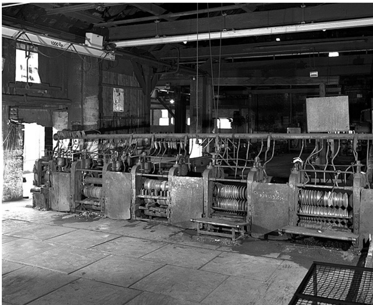
Laminage vu de trois quarts droit.
