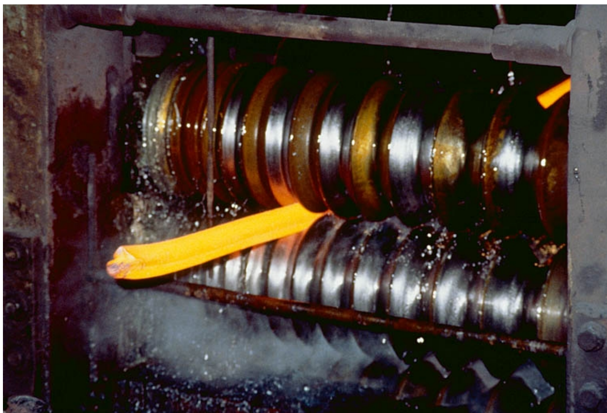
Laminoir : travail en cage de dégrossis (détail).
