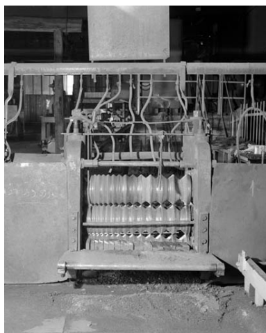
Cage du laminoir : dégrossis. Phot. Yves Sancey IVR43_19923900897X
