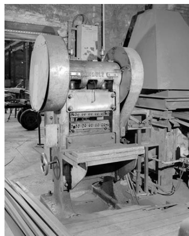
Atelier de préparation des soies : marteau-pilon Renault. Phot. Yves Sancey IVR43_19923900908X
