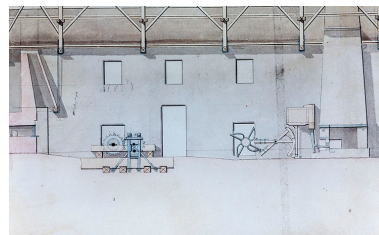
Coupe sur la longueur de la forge [détail de la refenderie, du laminoir et du soufflet]. Phot. Daniel Lebée IVR43_19933900046XA
