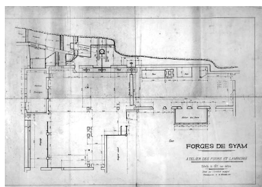
Forges de Syam. Atelier des fours et laminoirs. Phot. Jérôme Mongreville, Phot. Charles-Alfred Schacre IVR43_19923900824V
