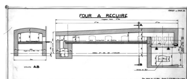
Four à recuire [coupes]. Phot. Jérôme Mongreville IVR43_19923900831V
