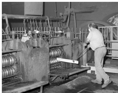
Laminoir : billeterie en cage de dégrossis. Phot. Yves Sancey IVR43_19923900947X
