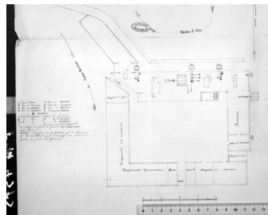
Plan des forges de Syam appartenant à Madame Veuve Jobez [...], détail de l'usine. Phot. Daniel Lebée IVR43_19933900050X
