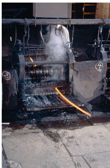
Laminoir : travail en cage de dégrossis (détail). Phot. Yves Sancey IVR43_19943900059ZA
