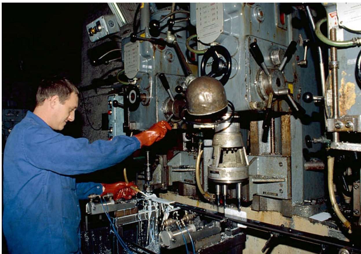
Atelier de parachèvement.
