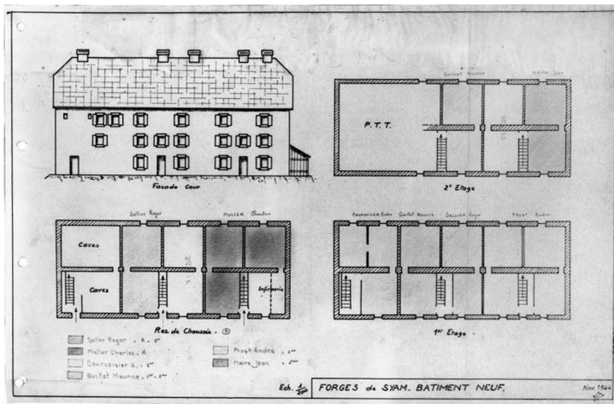
Forges de Syam. Bâtiment neuf [logement d'ouvriers et bureau de poste].
