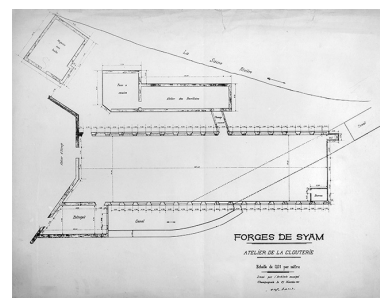
Forges de Syam. Atelier de la clouterie. Phot. Jérôme Mongreville, Phot. Charles-Alfred Schacre IVR43_19923900825V
