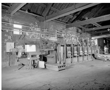
Four vu de trois quarts gauche. Phot. Yves Sancey IVR43_19923900892X
