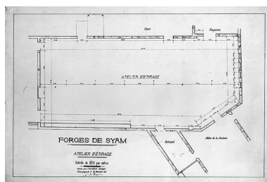
Forges de Syam. Atelier d'étrirage. Phot. Jérôme Mongreville, Phot. Charles-Alfred Schacre IVR43_19923900827V
