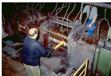
Laminoir : travail en cage de dégrossis. Phot. Yves Sancey IVR43_19943900046ZA
