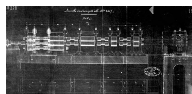
Ensemble d'un train petit mill. Dtre 260 m/m. Phot. Jérôme Mongreville, Autr. Chavanne Brun Frères IVR43_19923900838V
