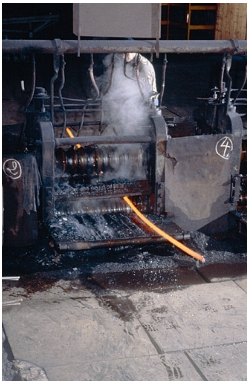
Laminoir : travail en cage de dégrossis (détail).
