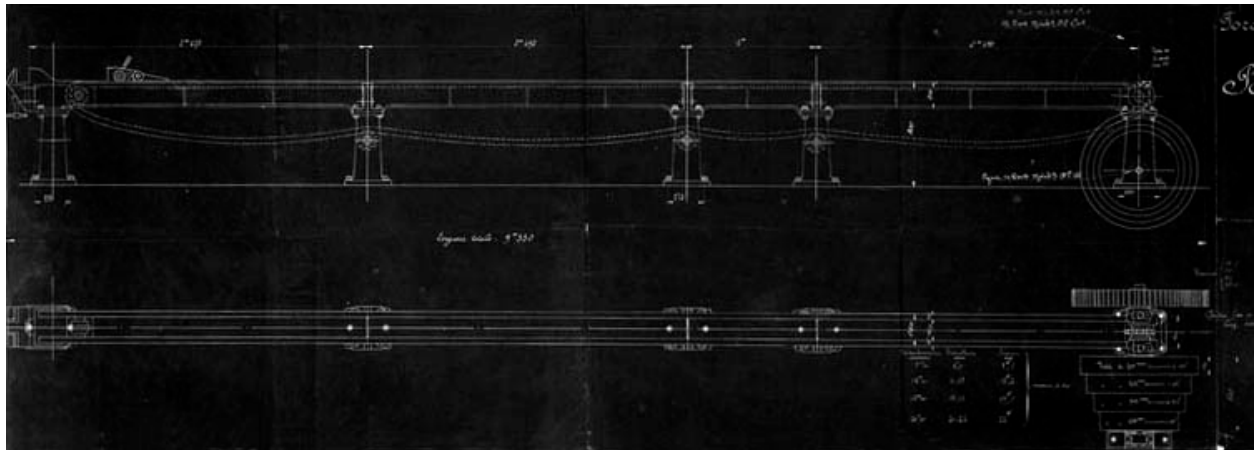
Forges de Syam. Banc à étirer de 5 tonnes. Ensemble.
