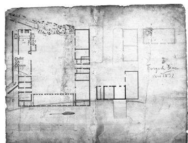
Plan de distribution de l'usine et de logements ouvriers. Phot. Jérôme Mongreville IVR43_19923900836V
