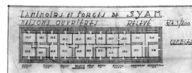
Laminoirs et Forges de Syam. Maisons ouvrières. Relevé. Combles. Phot. Jérôme Mongreville IVR43_19923900833V
