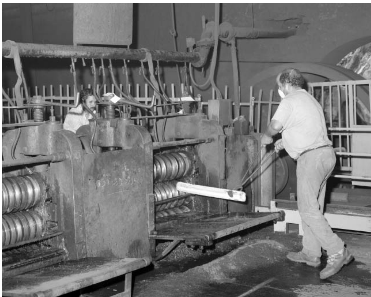
Laminoir : billeterie en cage de dégrossis.
