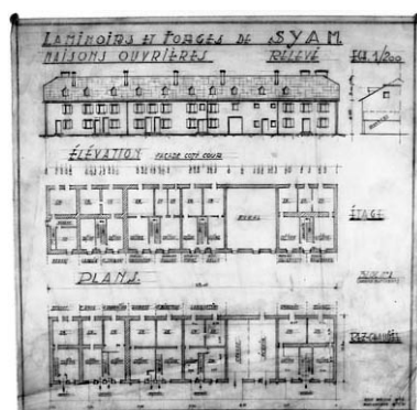
Laminoirs et Forges de Syam. Maisons ouvrières. Relevé.
