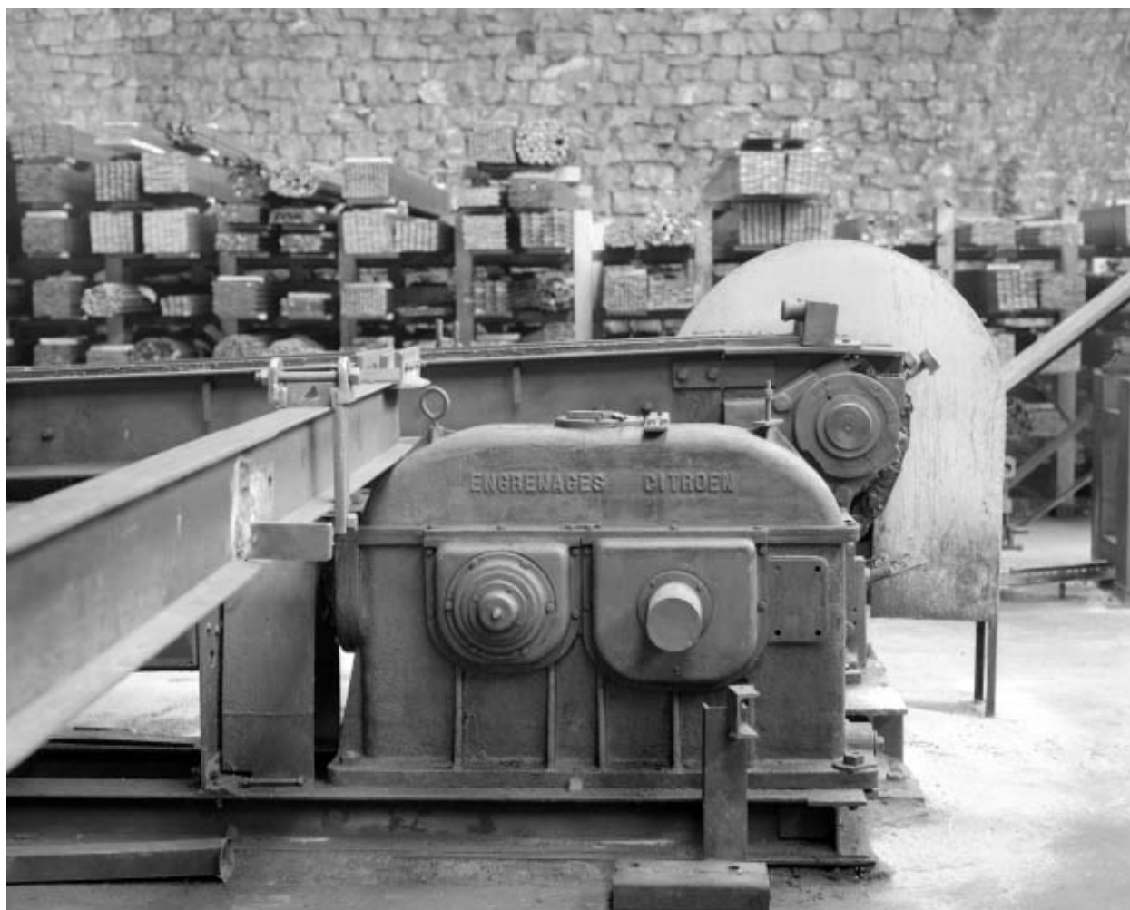
Banc d'étirage : système de transmission à engrenages Citroën.
