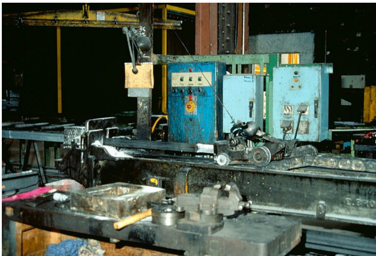
Atelier d'étirage : étirage d'une barre d'acier.
