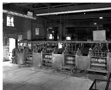
Laminoir vu de trois quarts droit. Phot. Yves Sancey IVR43_19923900896X
