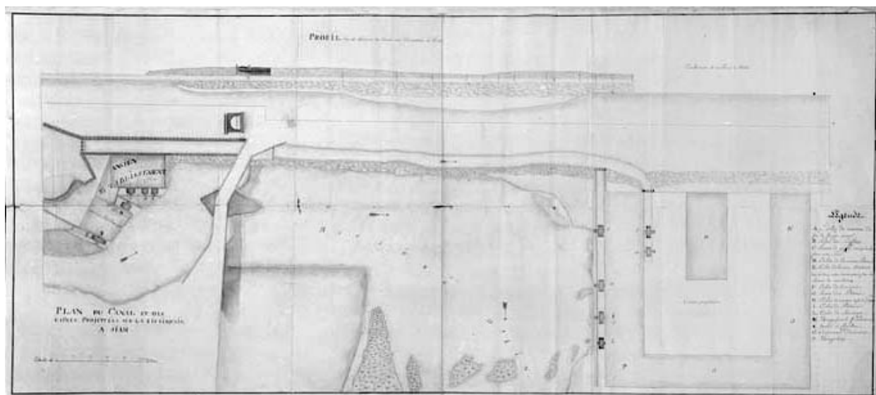
Plan du canal et des usines projetées sur la rivière d'Ain à Siam.
