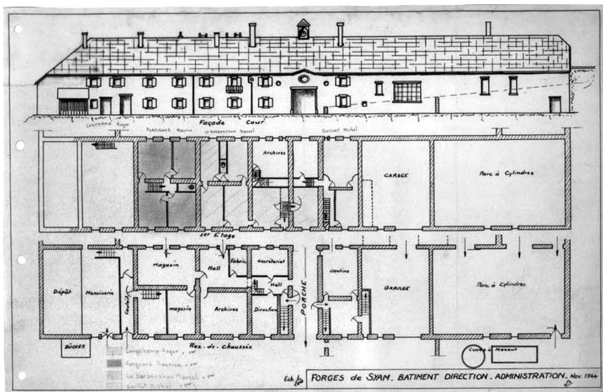
Forges de Syam. Bâtiment direction-administration.
