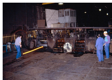
Laminoir : travail en cage de dégrossis. Phot. Yves Sancey IVR43_19943900061ZA
