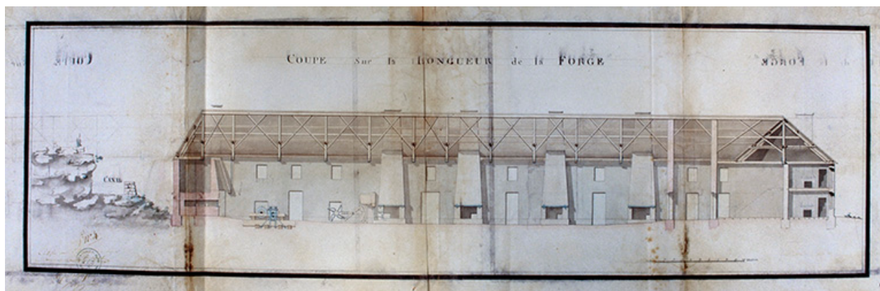
Coupe sur la longueur de la forge.
