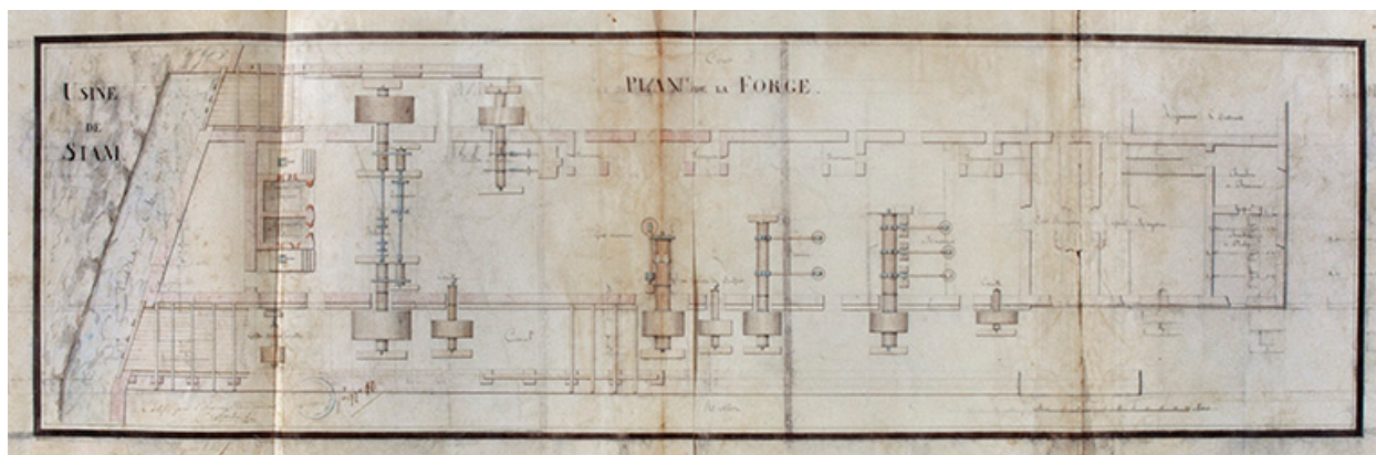
Plan de la Forge.
