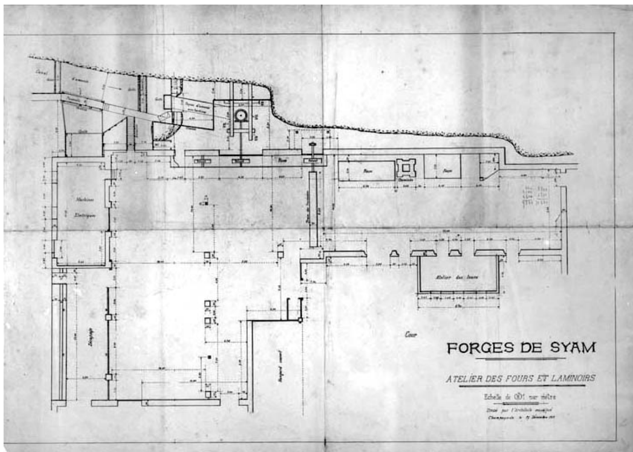
Forges de Syam. Atelier des fours et laminaires.
