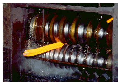
Laminoir : travail en cage de dégrossis (détail). Phot. Yves Sancey IVR43_19943900050ZA
