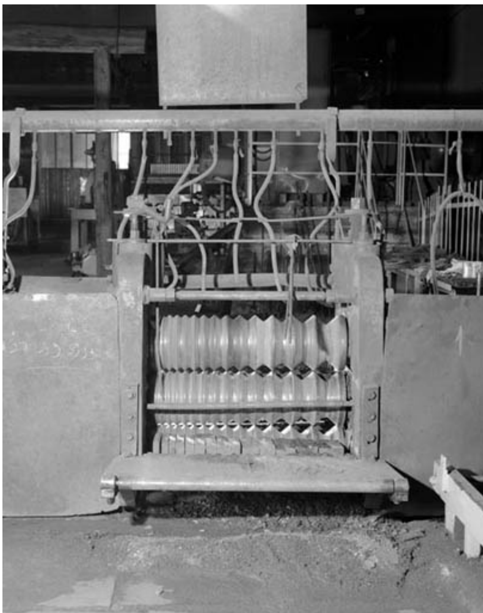
Cage du laminoir : dégrossis.
