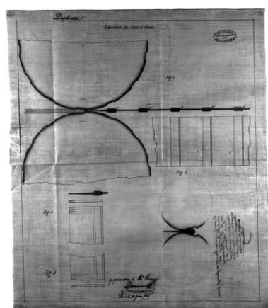
Fabrication des clous à ferrer [coupe de cylindres cannelés]. Phot. Jérôme Mongreville IVR43_19923900830V
