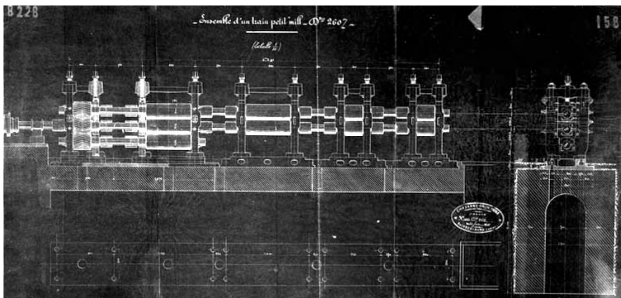
Ensemble d'un train petit mill. Dtre 260 m/m.
