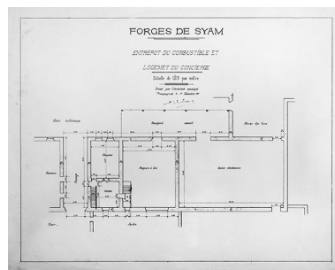
Forges de Syam. Entrepôt du combustible et logement du concierge. Phot. Jérôme Mongreville, Phot. Charles-Alfred Schacre IVR43_19923900828V
