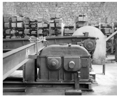
Banc d'étirage : système de transmission à engrenages Citroën. Phot. Yves Sancey IVR43_19923900915X
