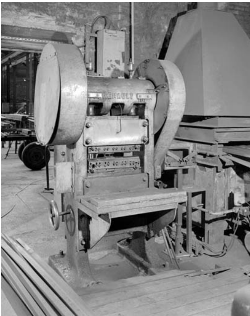
Atelier de préparation des soies : marteau-pilon Renault.
