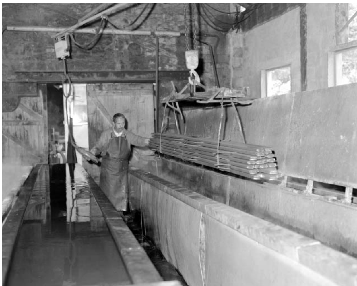
Atelier de décapage : déplacement des barres.
