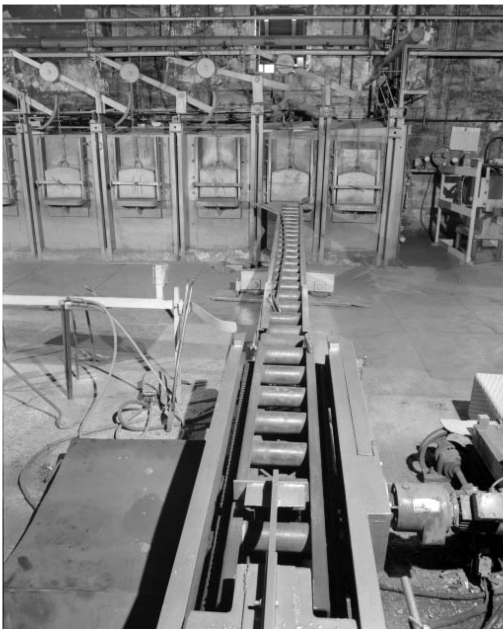
Four et transporteur à rouleaux.
