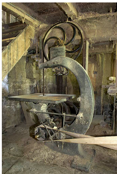
Rez-de-chaussée. Scie à ruban J. Guillet - Egré et Cie. Phot. Jérôme Mongreville IVR43_20057000251NUCA
