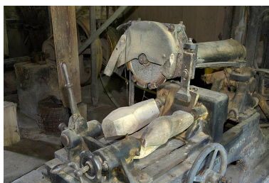
Rez-de-chaussée. Tour à reproduire Bonneau & Schwartz et Cie. Phot. Jérôme Mongreville IVR43_20057000250NUCA
