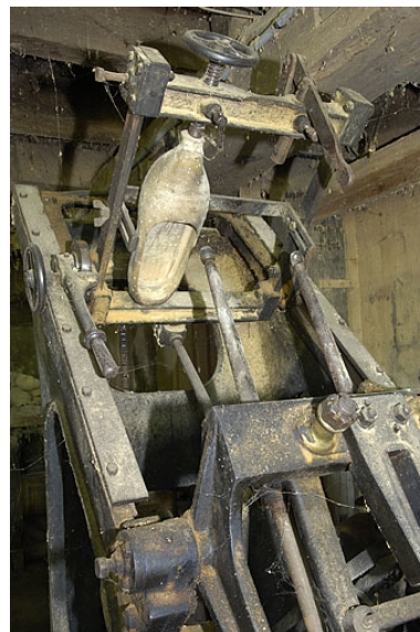
Rez-de-chaussée. Tour à cuillères (videuse) Bonneau & Schwartz et Cie. Détail de la partie supérieure. Phot. Jérôme Mongreville IVR43_20057000253NUCA
