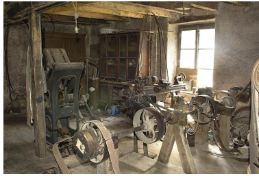
Premier étage. Vue de l'atelier depuis l'ouest. Au premier plan : banc d'affûtage. Phot. Jérôme Mongreville IVR43_20057000259NUCA
