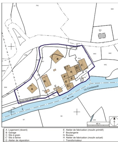
Plan-masse et de situation. Extrait du plan cadastral numérisé, 2008, section B, 1:1250. Source : Direction générale des Finances Publiques - Cadastre ; mise à jour : 2008. Dess. André Céréza IVR43_20087000246NUDA
