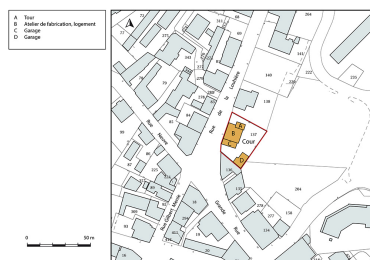
Plan-masse et de situation. Extrait du plan cadastral, 2018, section AE, 1/1 000. Dess. Bertrand Turina IVR43_20182501395NUDA
