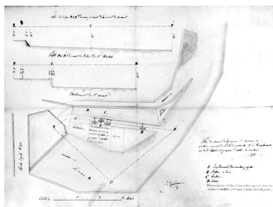
Plan du cours de la rivière de Cuisance à Arbois, auprès du Pont de Couturette et de l'emplacement où le sieur Bechet se propose d'établir ses moulins. Phot. Jérôme Mongreville IVR43_19963901765V
