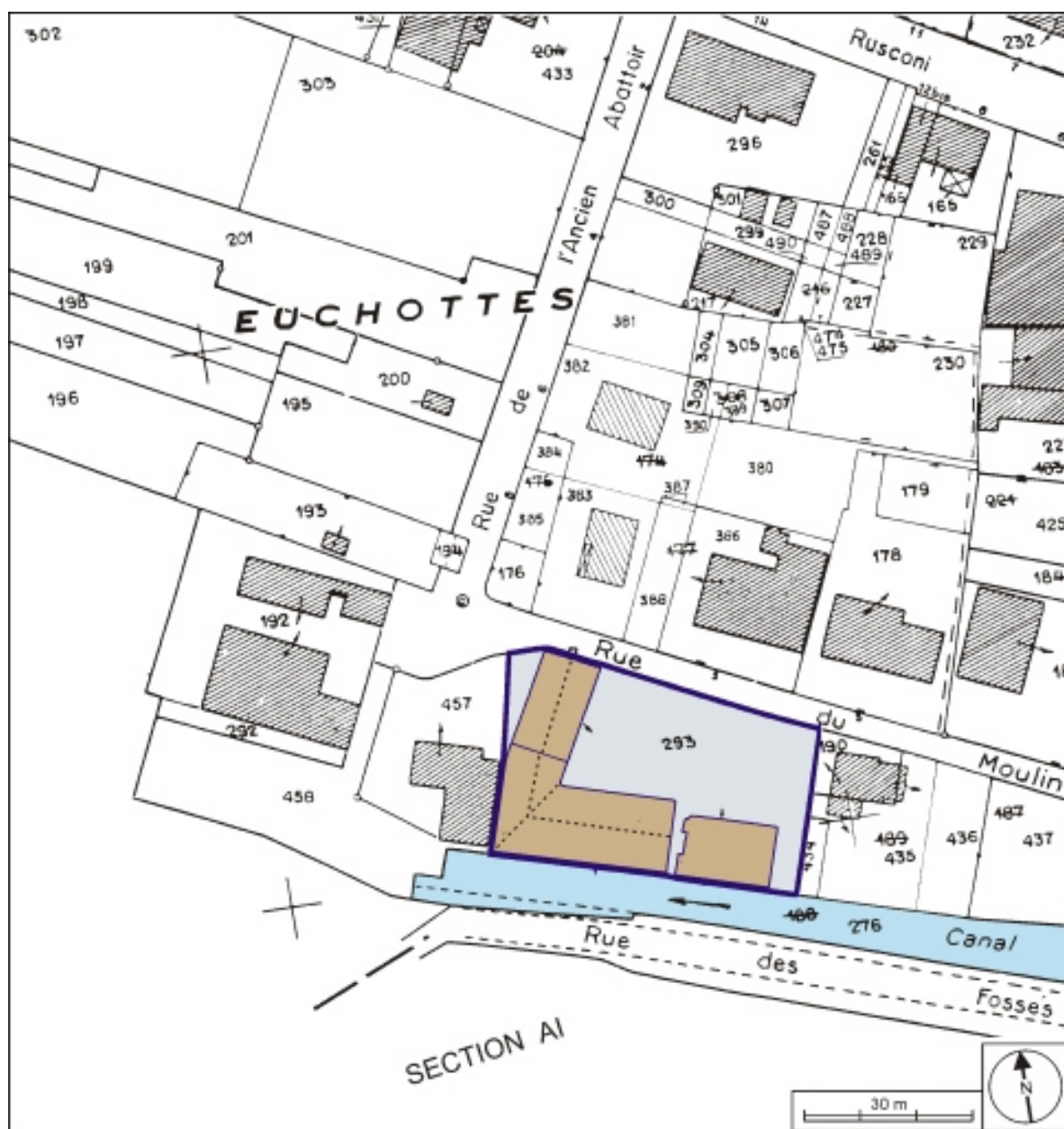
Plan-masse et de situation. Extrait du plan cadastral, 1984, section AB, 1:1000.
