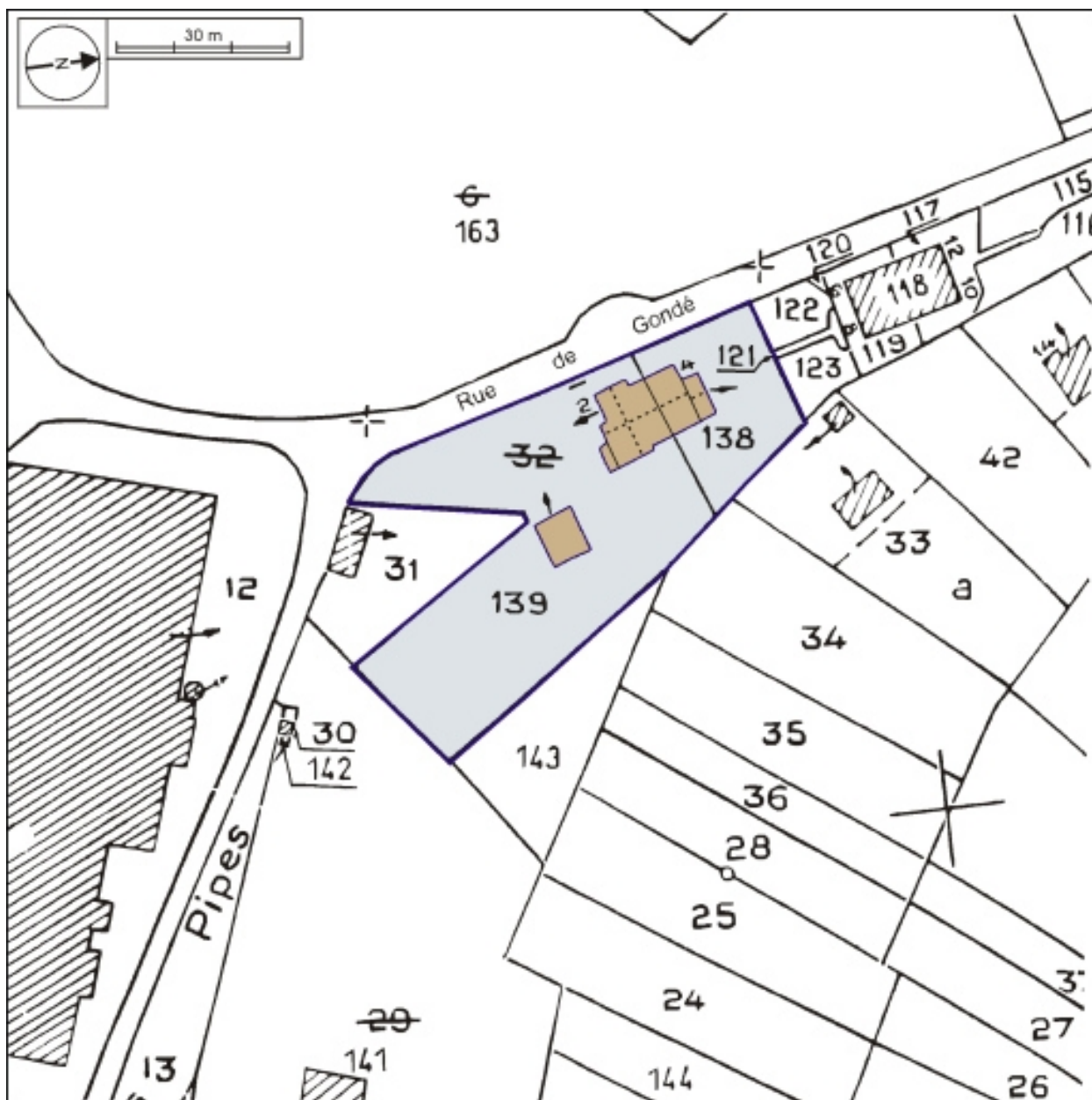
Plan-masse et de situation. Extrait du plan cadastral, 1982, section ZN, 1:2000 agrandi à 1:1000.
