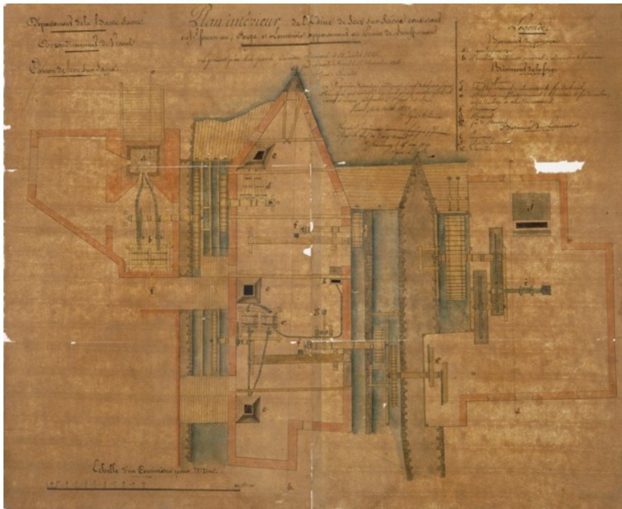
Plan intérieur de l'usine de Scey-sur-Saône consistant en haut fourneau, forges et laminoir [...].
