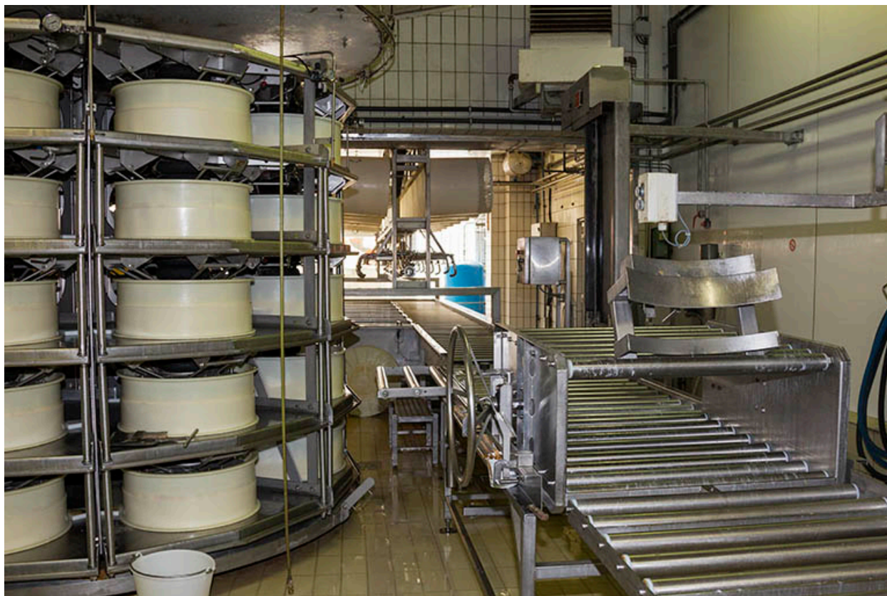
Installation de pressage et convoyeur.
