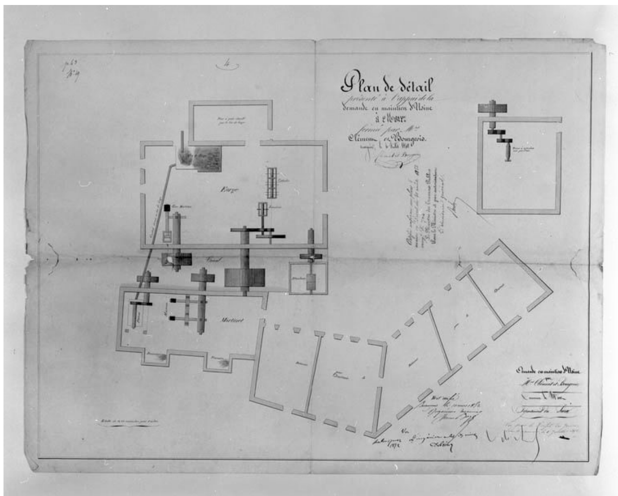
Plan de détail présenté à l'appui de la demande en maintien d'Usine à Morez formée par Mrs Clément et Bourgeois [...]. Dessin, 1840. Echelle 1:100.
