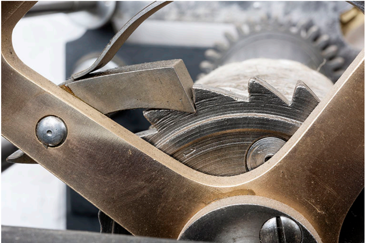
Mouvement, mécanisme des sonneries : détail du cliquet.
