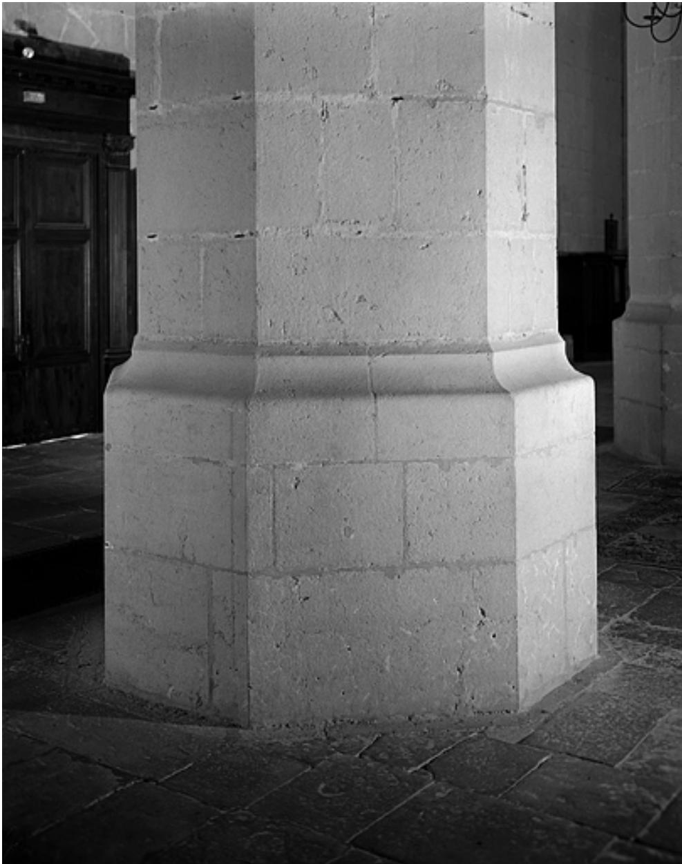
Base de la pile VS (vue verticale).
