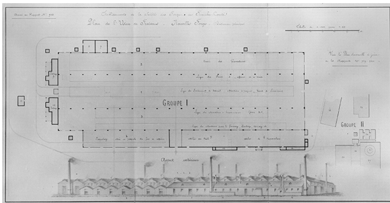
Etablissements de la Société des Forges de Franche-Comté. Plan de l'Usine de Fraisans. Nouvelle Forge. Bâtiment principal.
