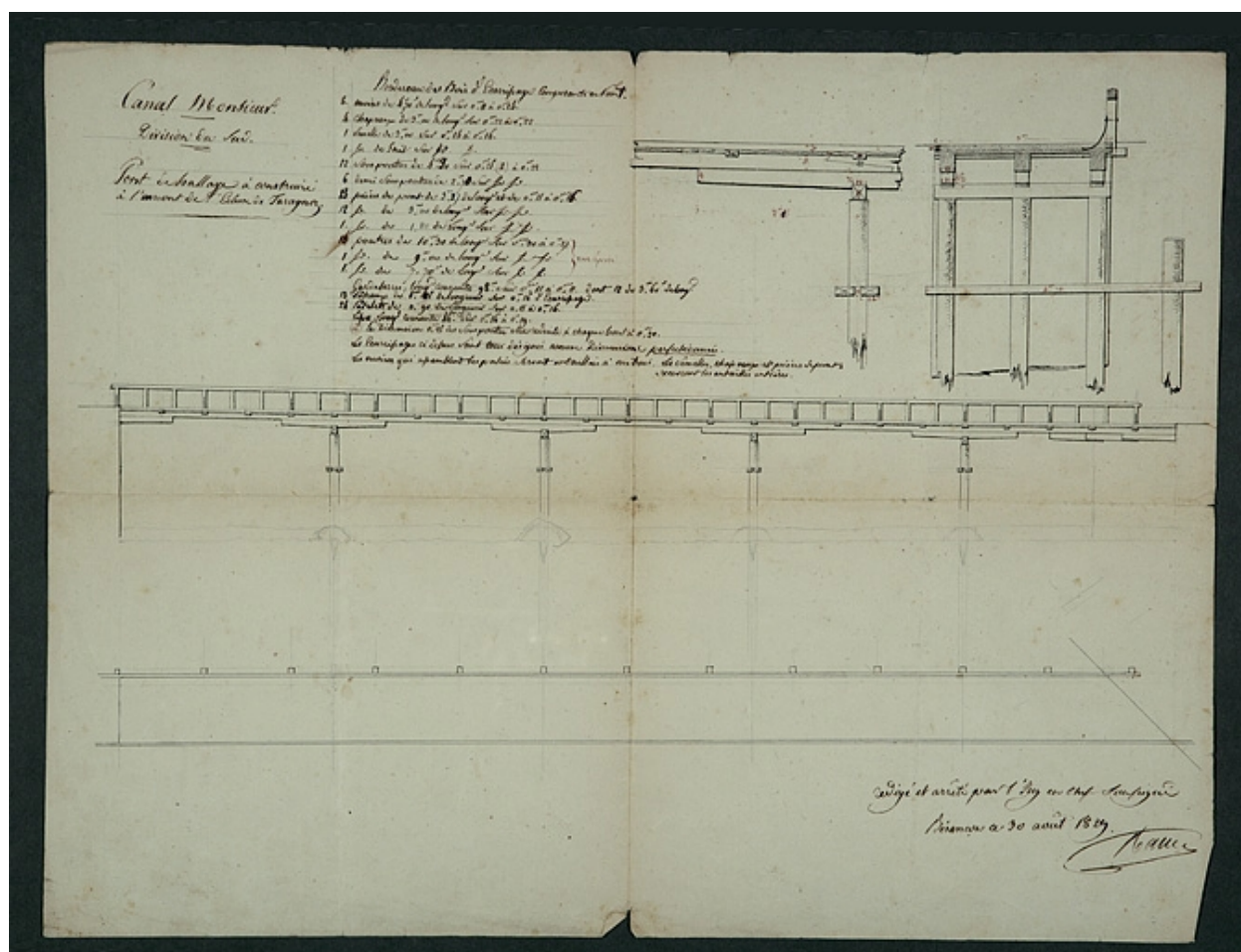
Pont de halage à construire à l'amont de l'écluse de Taragnoz, 1829.
