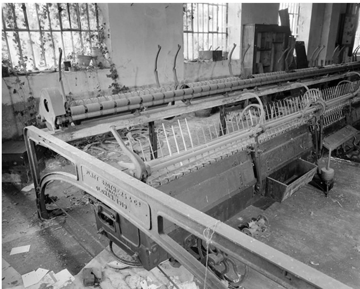
Extrémité du chariot du module de gauche.
