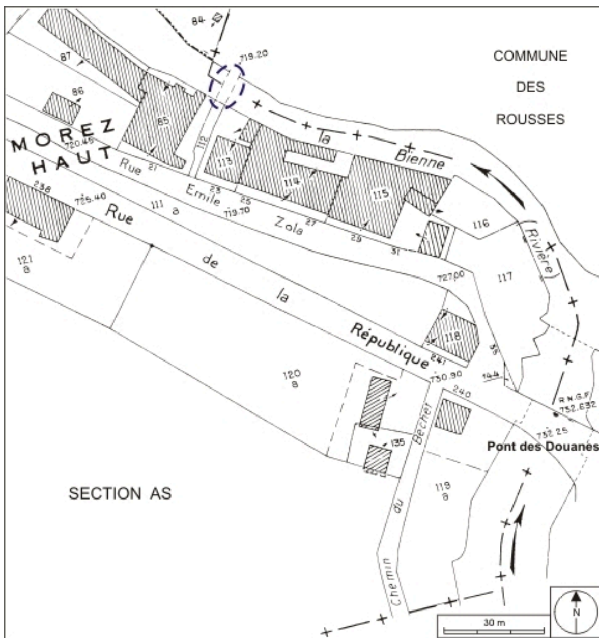
Plan de situation. Extrait du plan cadastral, 1980, section AK, échelle 1:1000.
