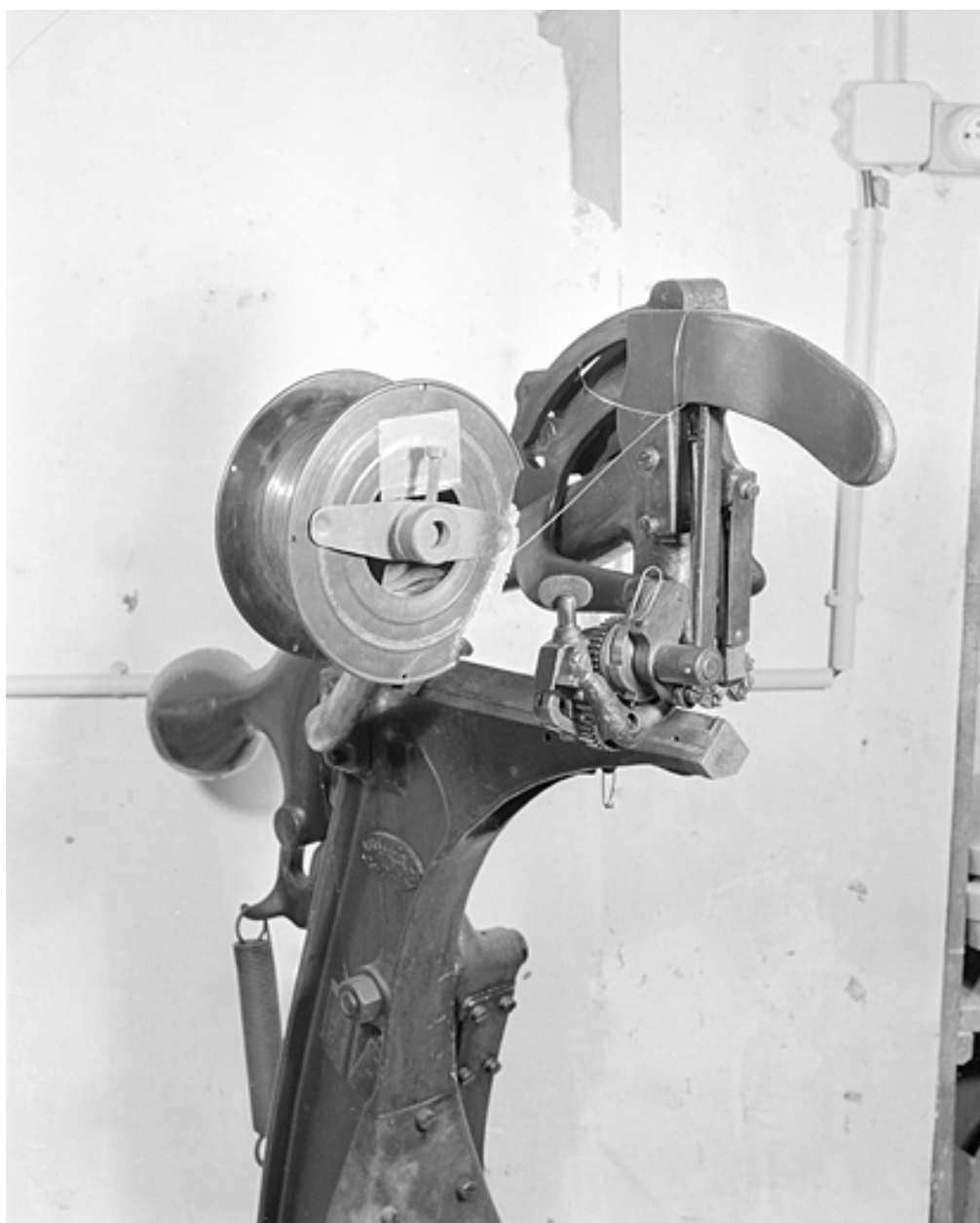
Détail du mécanisme d'agrafage.
