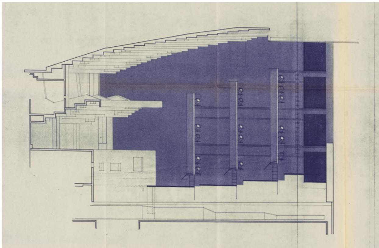
Ville de Nevers. Maison de la culture. Equipement scénique.SC 18. Plan du plafond de la salle et parois latérales [détail : parois]. 1968.
