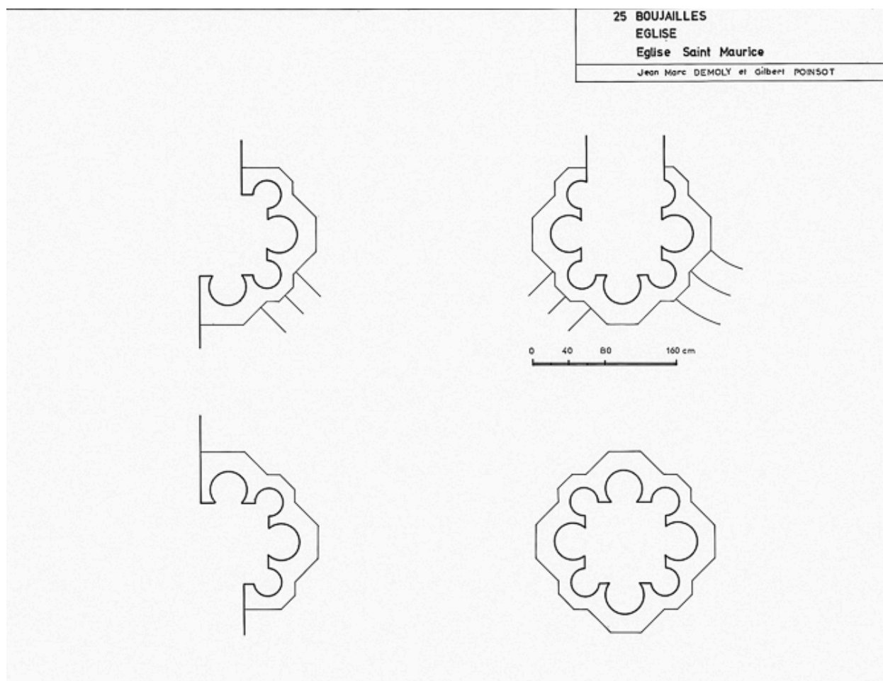
Plan des gros piliers : relevé-croquis J.M Demoly et G. Poinot, 1975.
