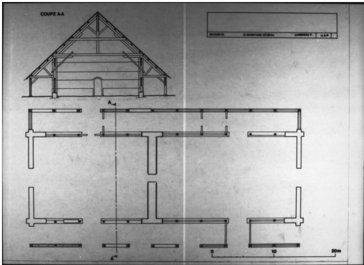
Plan et coupe de la halle à charbon. Relevé graphique, 1988, M. Brugier et F. Corbineau, échelle 1:1250.
