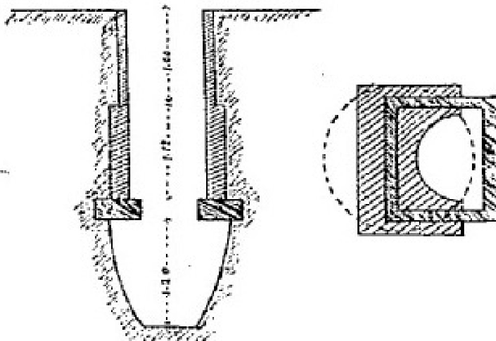
Fig. 63. — COUPE ET PLAN DU CAP- TAGE DE LA SOURCE DE MAIZIÈRES.
