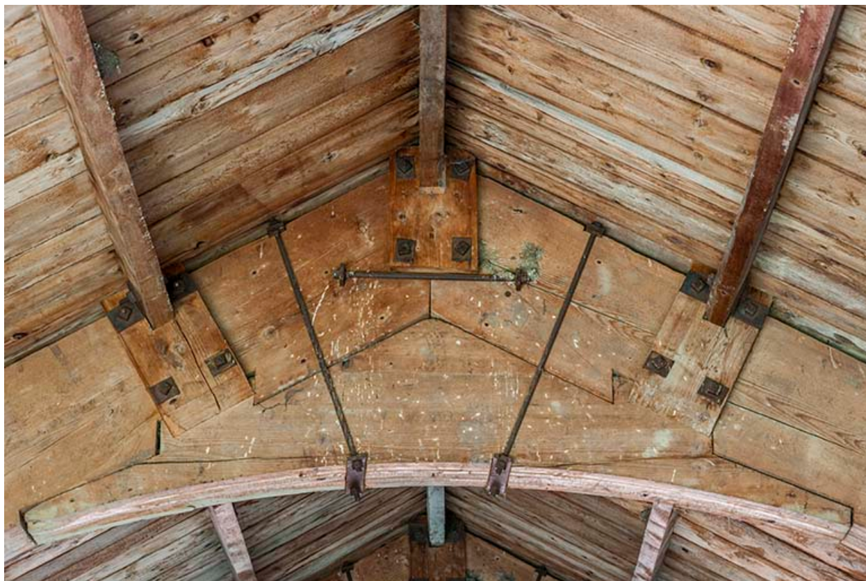
Détail de la jonction d'une ferme.
