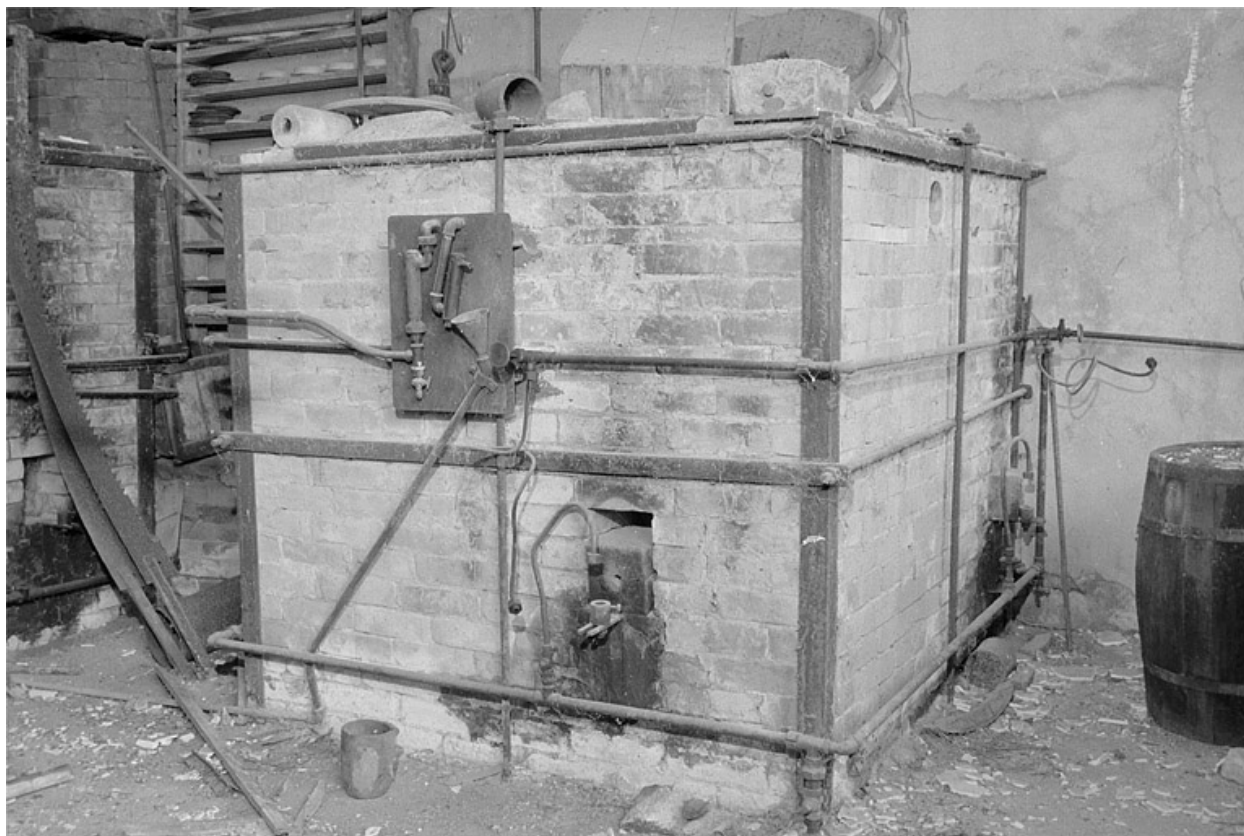
Four pour la fabrication des cylindres.
