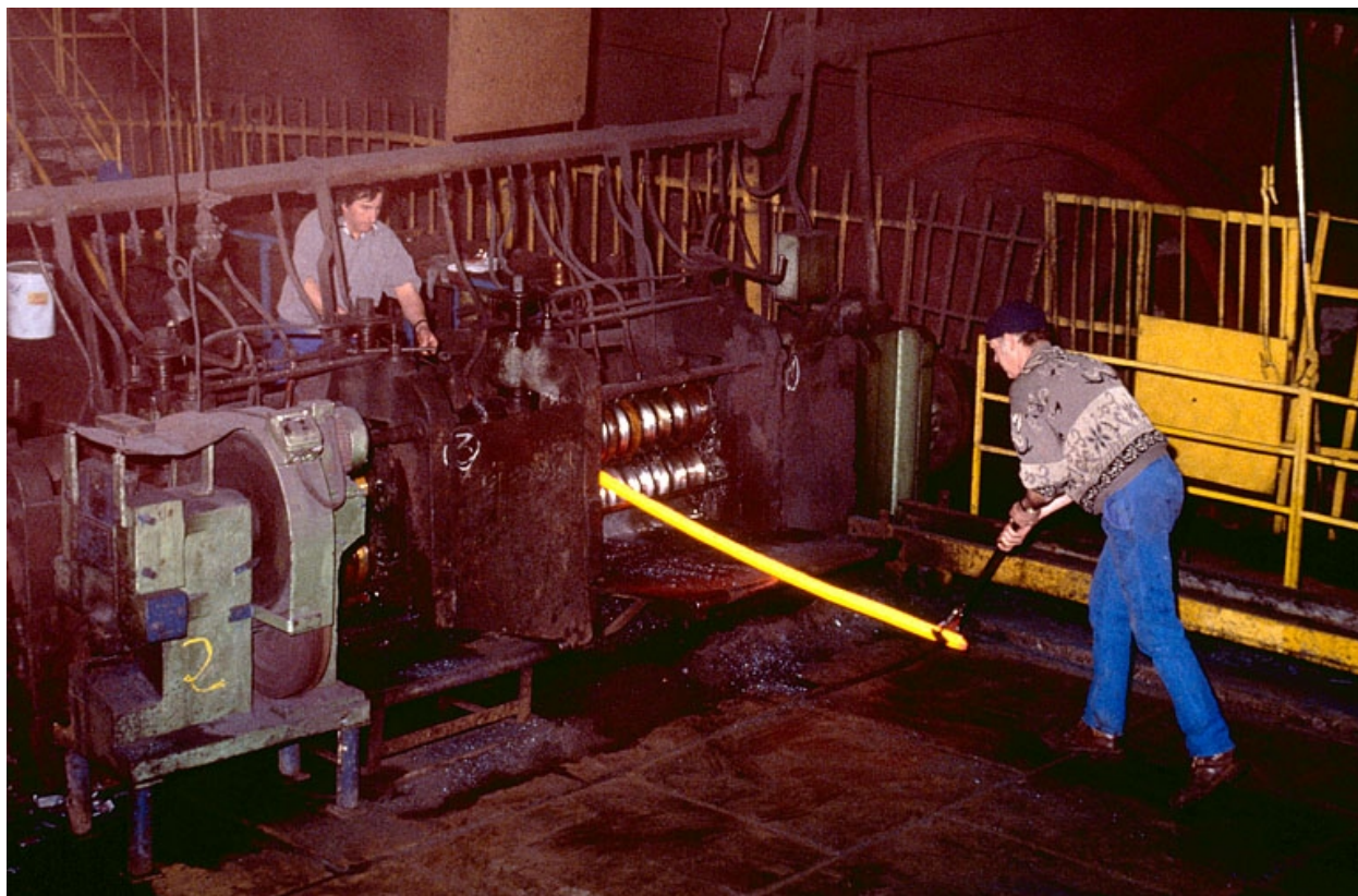
Laminoir : travail en cage de dégrossis.
