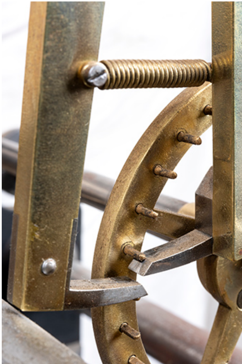
Mouvement, mécanisme des heures : échappement à chevilles (détail de l'ancre et des chevilles).
