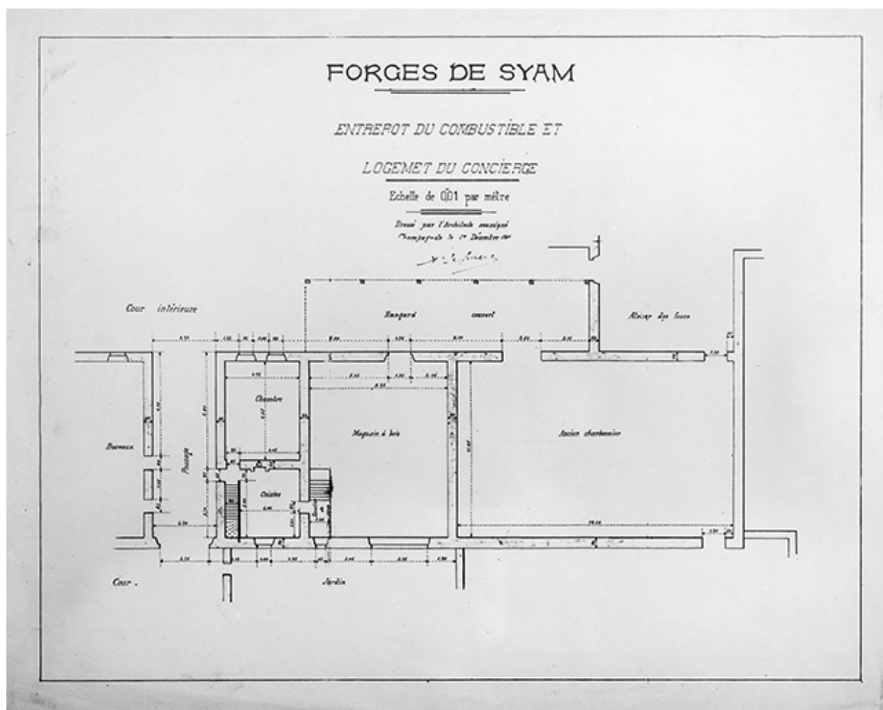
Forges de Syam. Entrepôt du combustible et logement du concierge.
