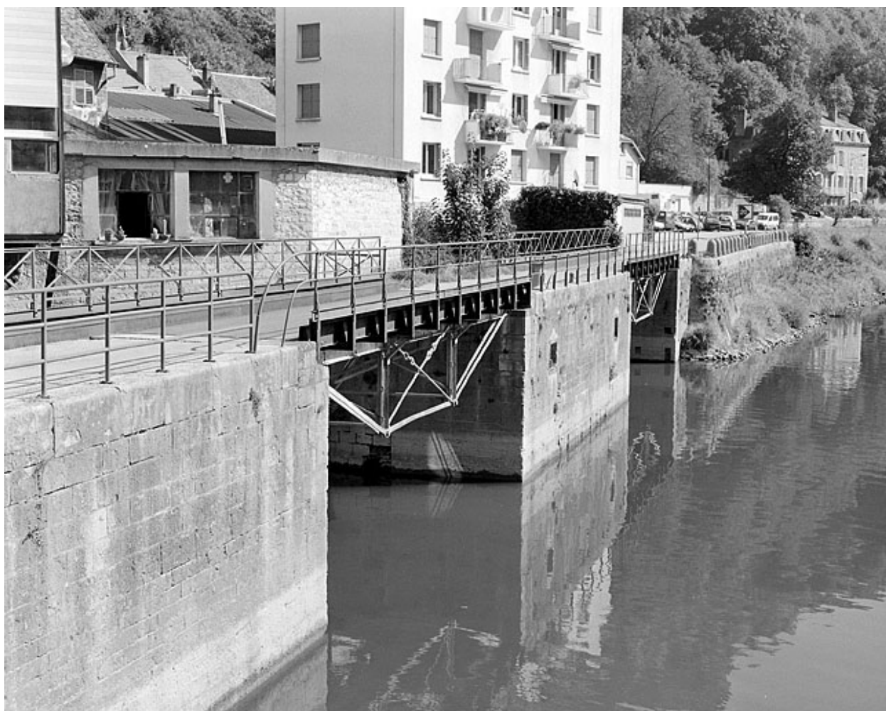
Ponts de halage sur les canaux de fuite de l'usine.
