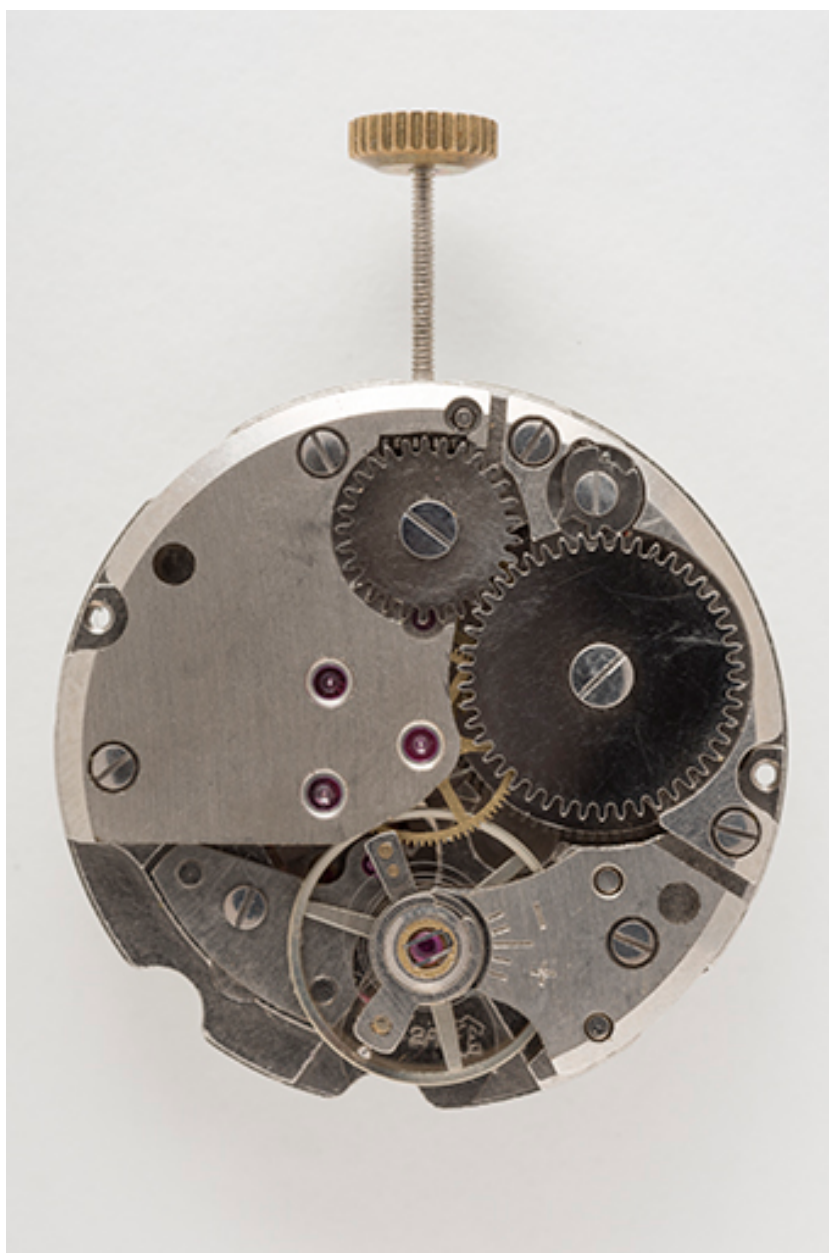
Mouvement FE 140-2A, vu côté pont.
