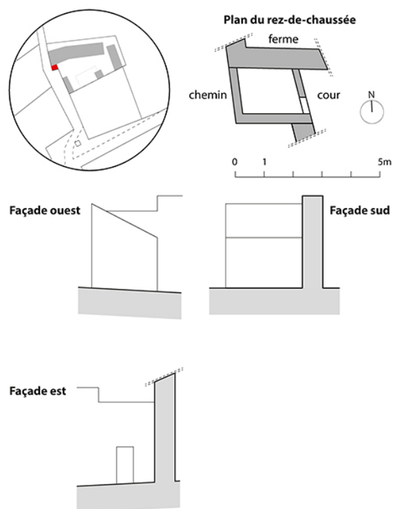
Ferme de Vaufron, Saint-Père (89) : toit à porcs
