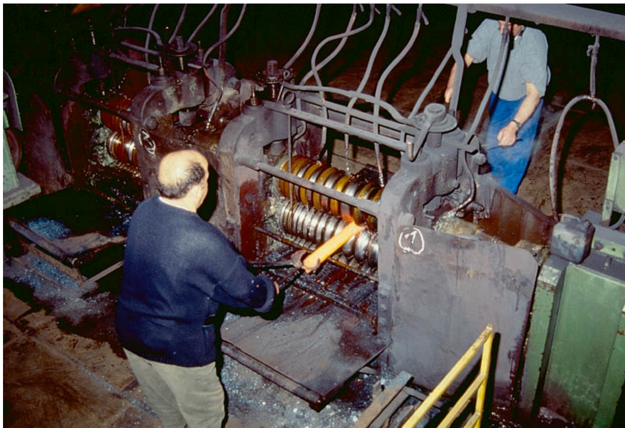
Laminoir : travail en cage de dégrossis.
