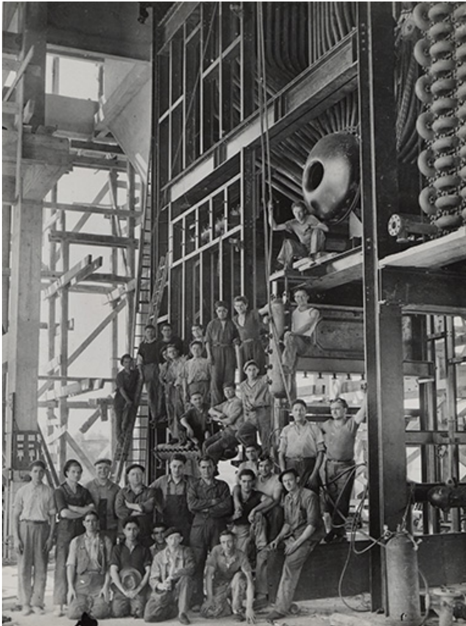
Construction de la centrale thermique. Equipe d'ouvriers.
