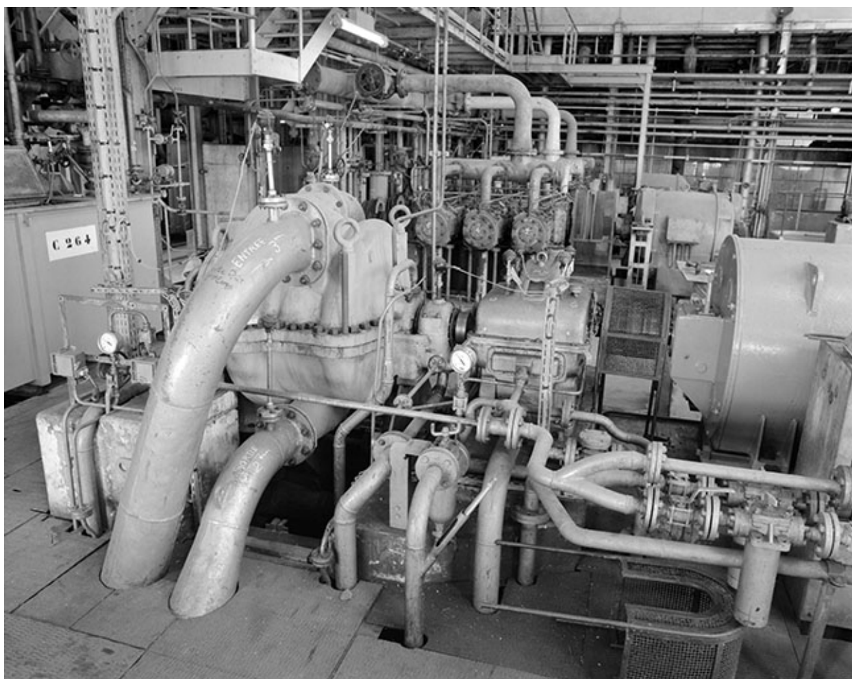
Usine d'électrolyse, Salle 3 : détail du compresseur Rateau et du variateur SACM de la soufflante à chlore.
