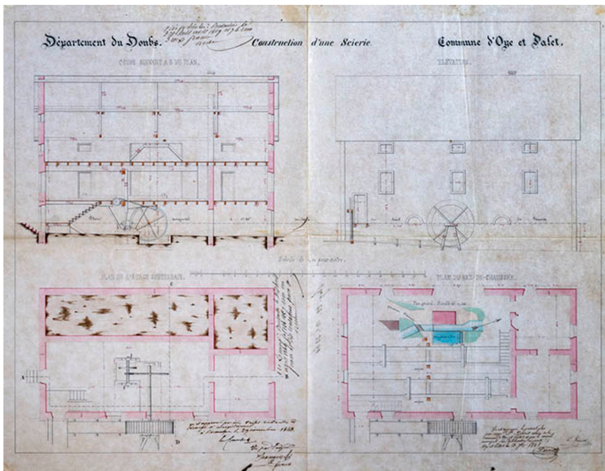
Construction d'une scierie [Plans, élévation et coupe], 1848.
