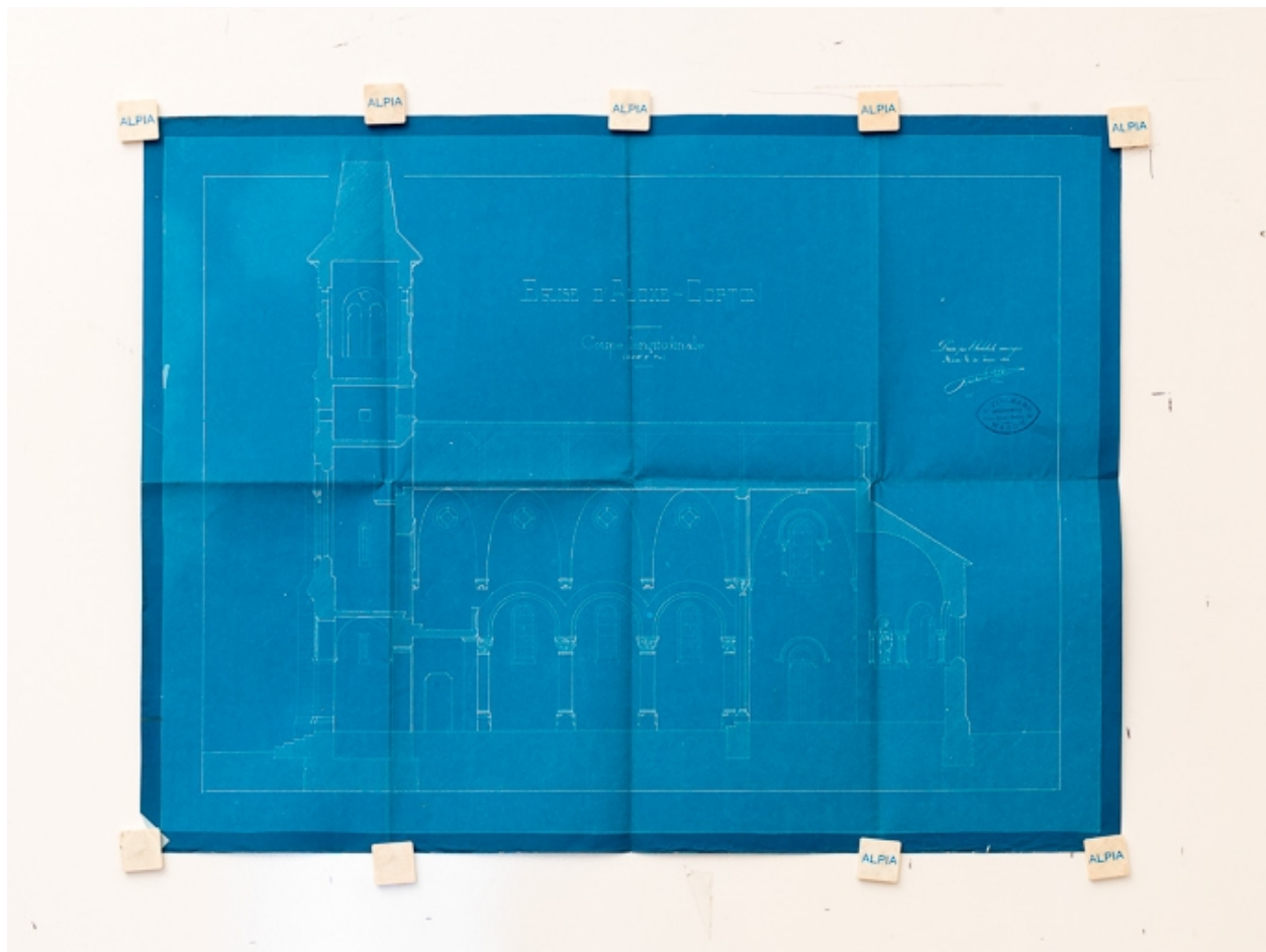
Coupe longitudinale de l'église d'Aloxé-Corton. Plan bleu dressé par l'architecte Pinchard le 30 juin 1888 (Archives communales, Aloxé-Corton).
