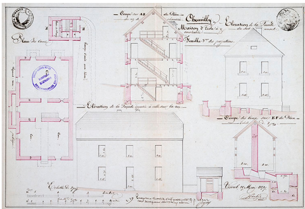
Plans de la maison d'école à construire, 1851
