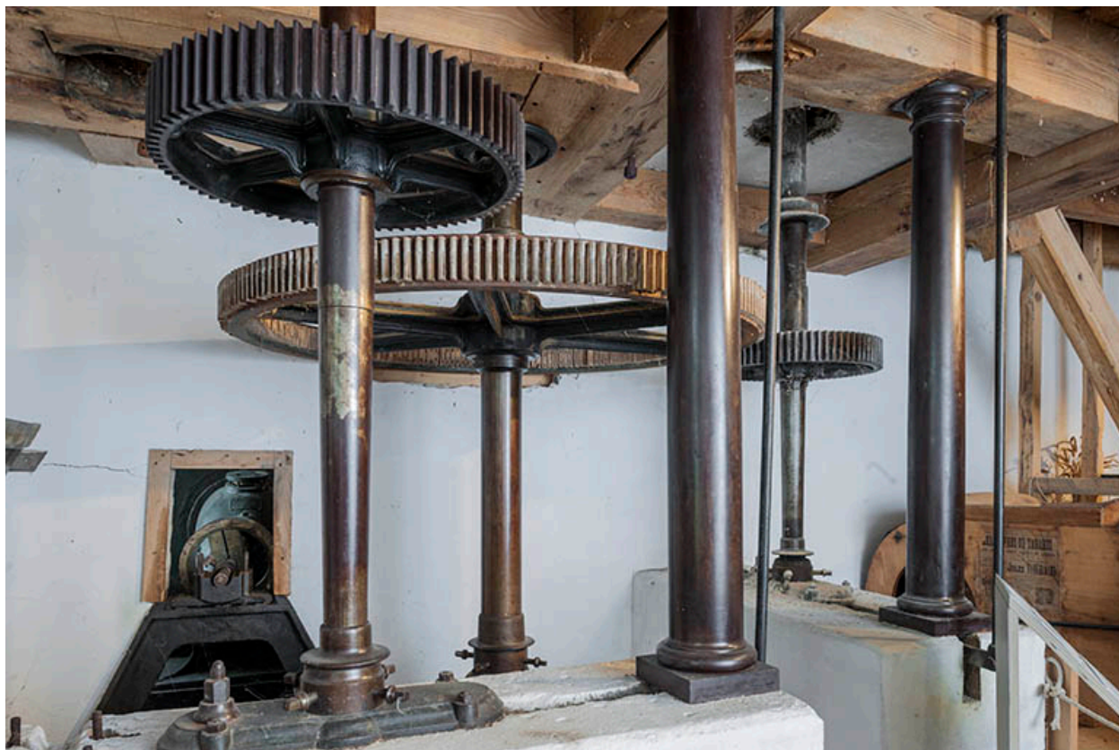
Rez-de-chaussée. Détail des transmissions et des colonnes du beffroi.
