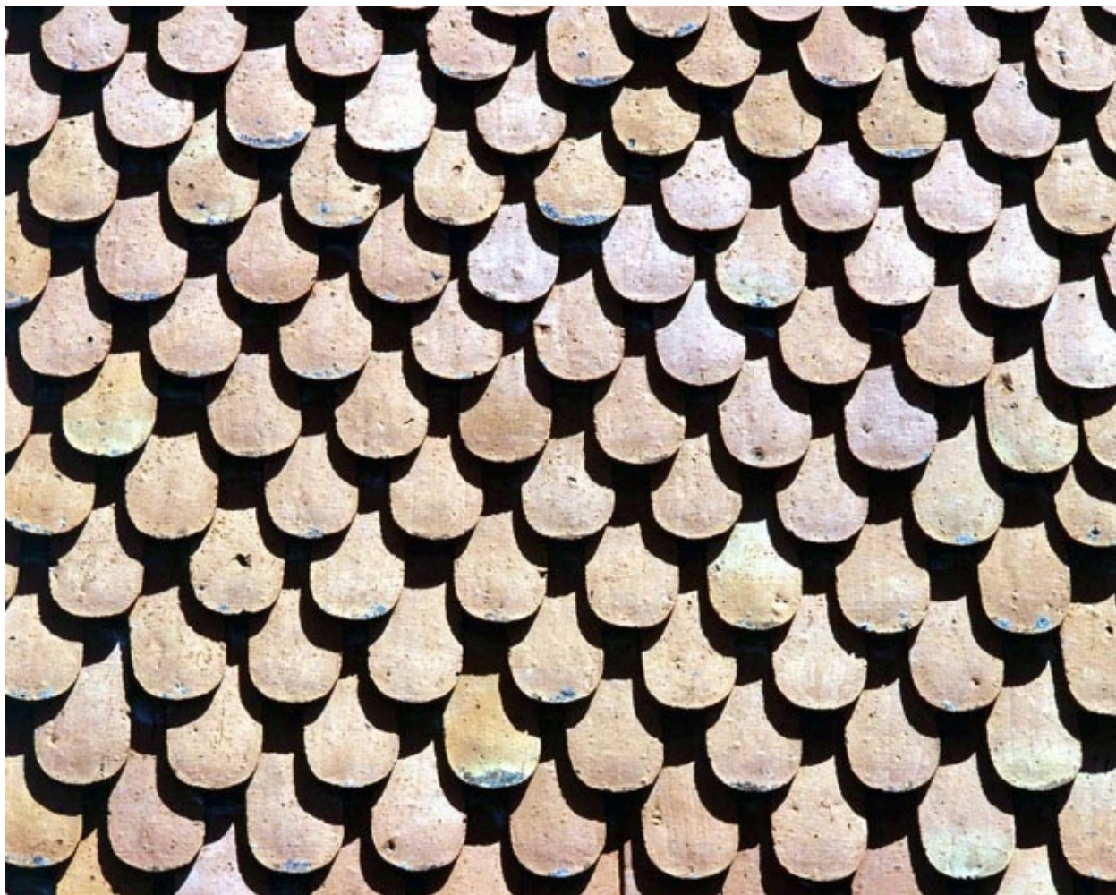
Essentage de tuiles écaille protégeant un mur (ferme aux Près de Valfin, à Saint-Claude).
