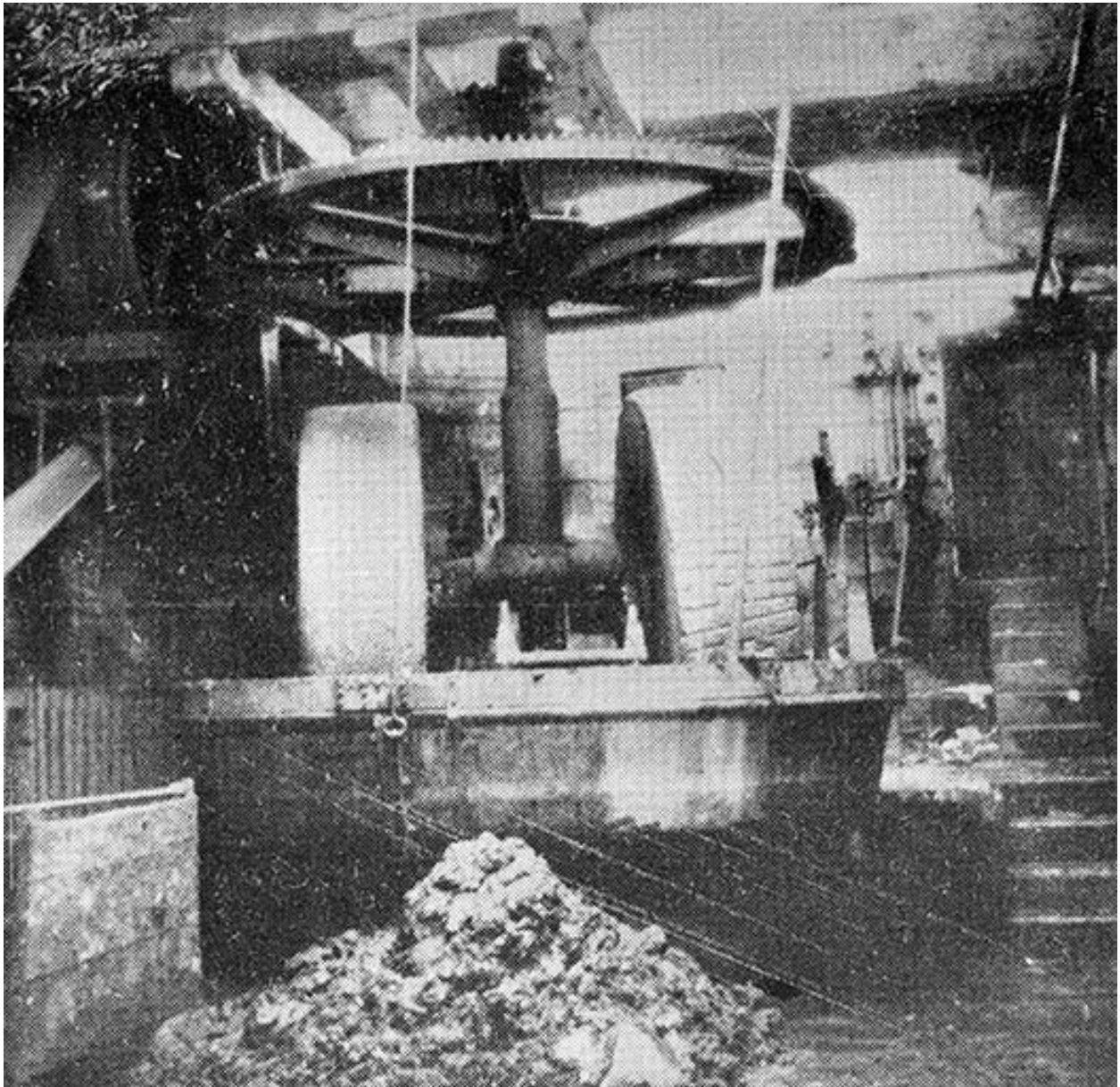
Meules d'écrasement de la pâte.
