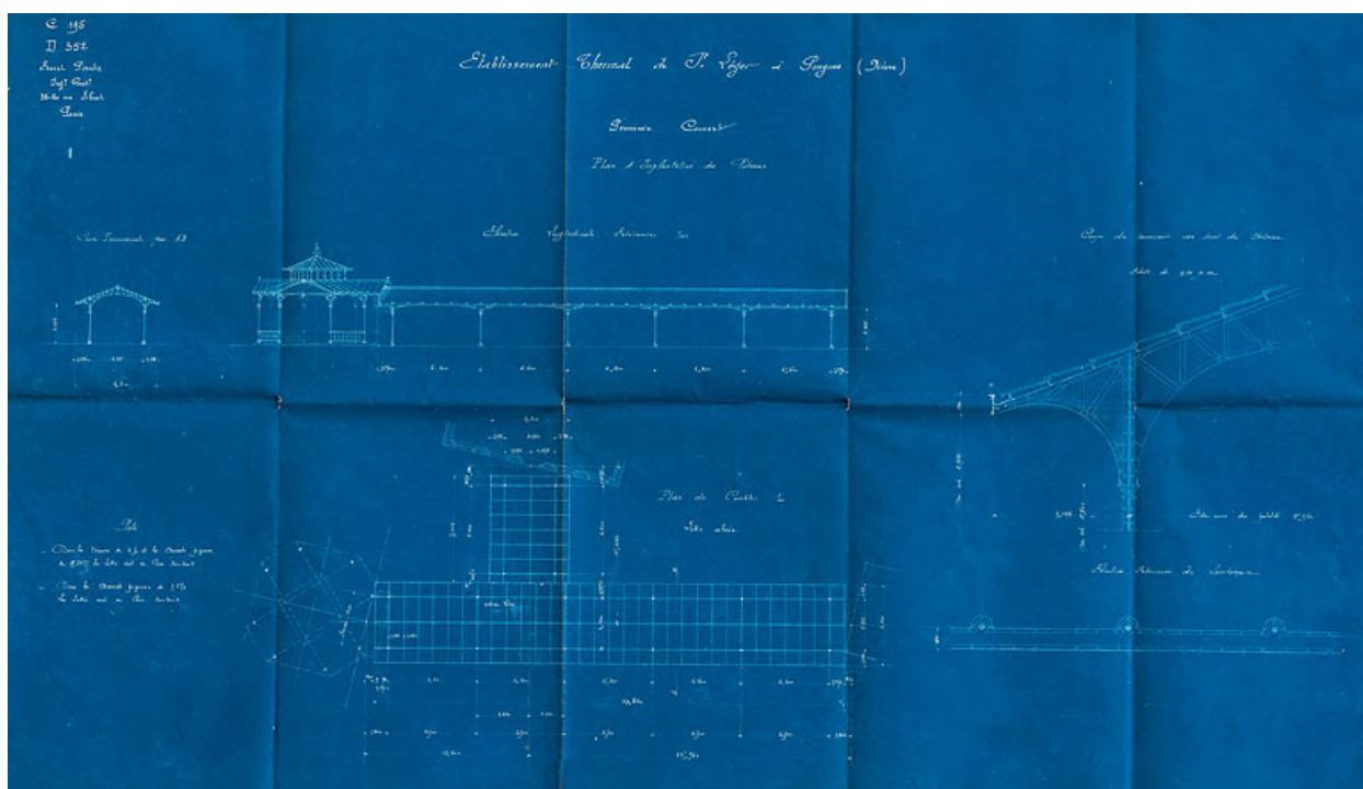
Promenoirs d'Ernest Pantz (1895) : plan, coupe et élévation.
