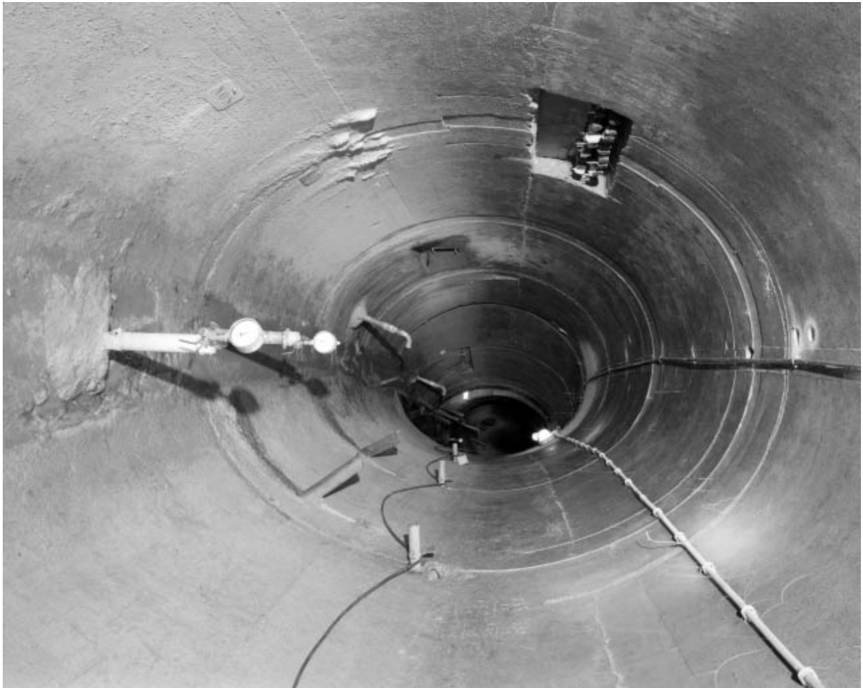
Système d'auscultation du barrage : réseaux piézométrique et de drainage.
