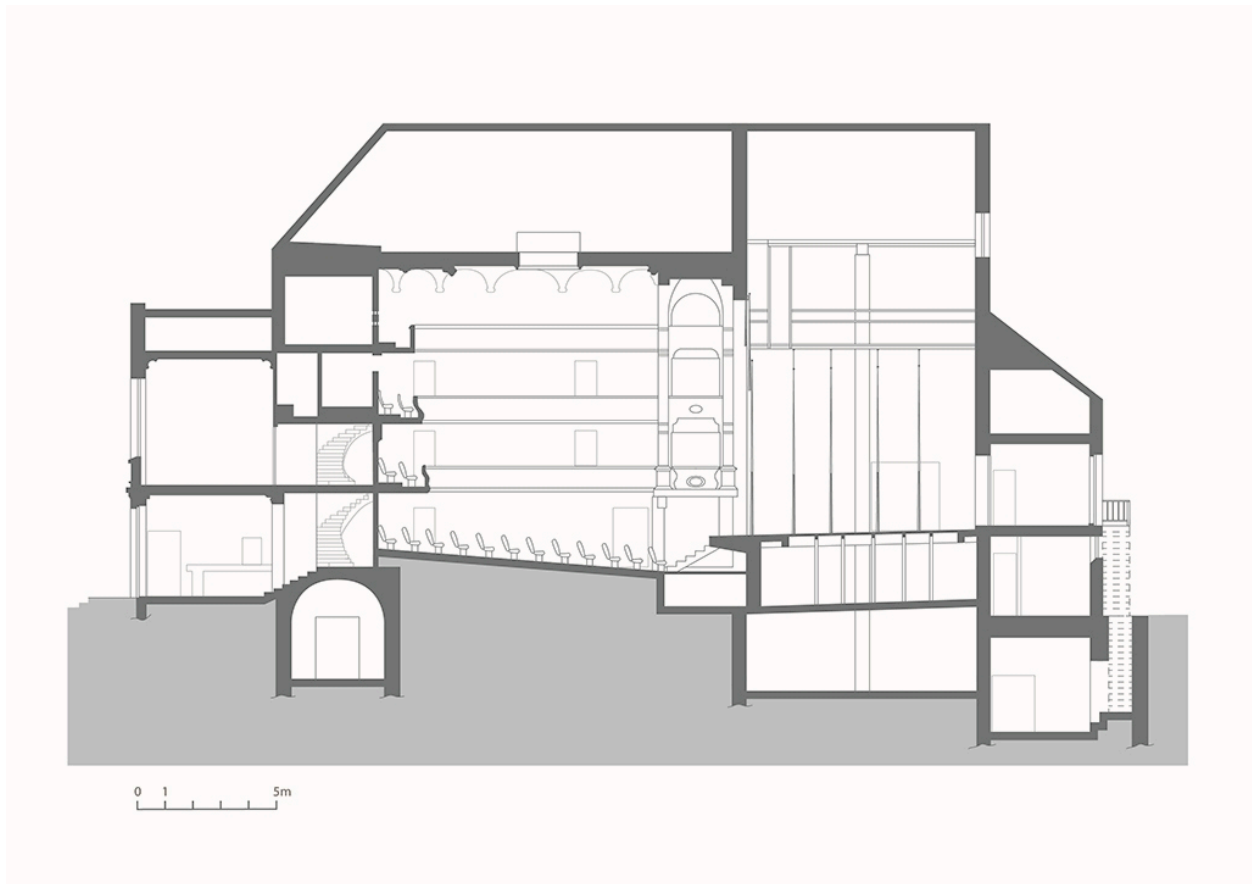
Coupe longitudinale. D'après une coupe de Jérôme Sabre.
