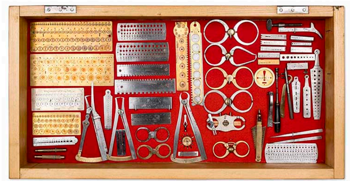
Outils produits dans la commune (collection René Laithier, mairie des Gras) : calibres, filières, huit-chiffres, bancs à river, etc.
