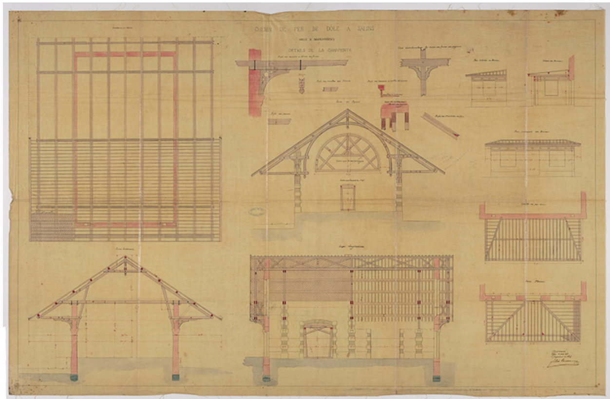
Chemins de fer de Dole à Salins. Halle à marchandises, 1855.
