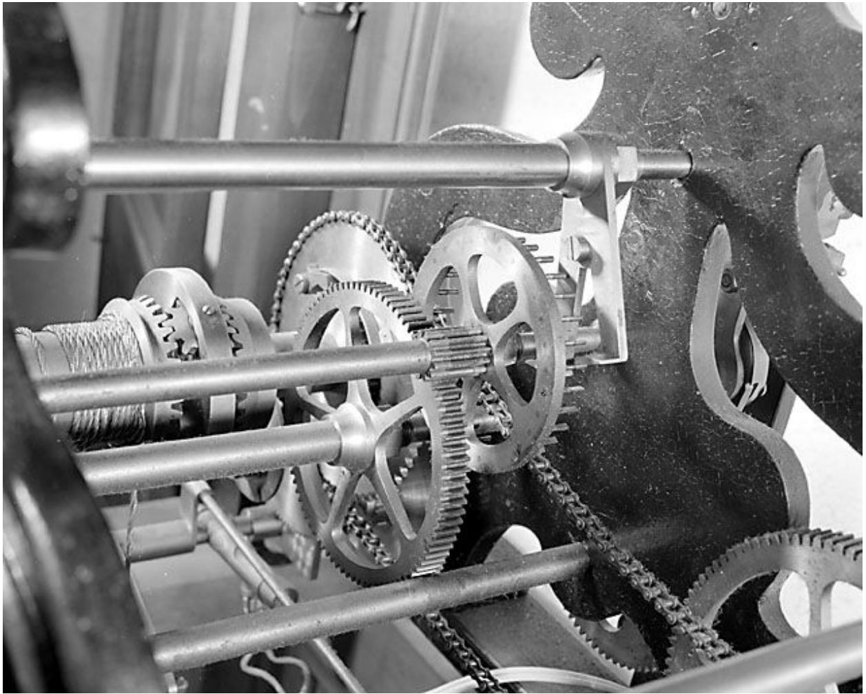
Echappement à ancre.
