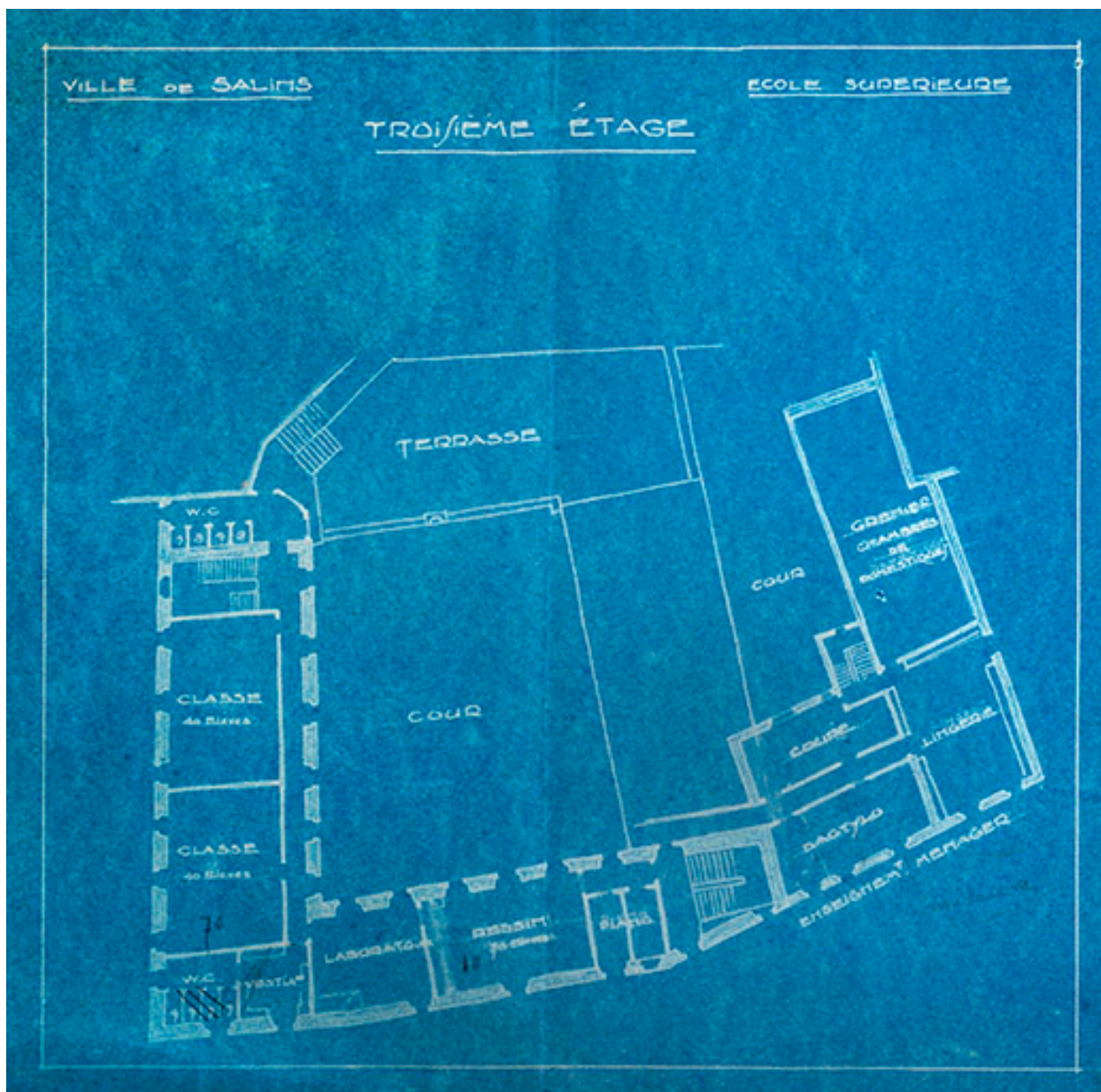
Projet d'aménagement de l'école Voltaire en école primaire supérieure. Plan du troisième étage, s.d. [1921].
