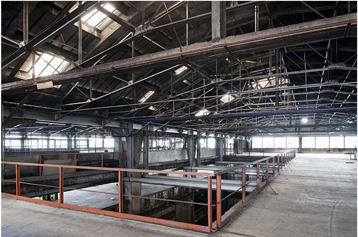
Entrepôt de stockage de véhicules (201) : voûte segmentaire et sa charpente métallique.
