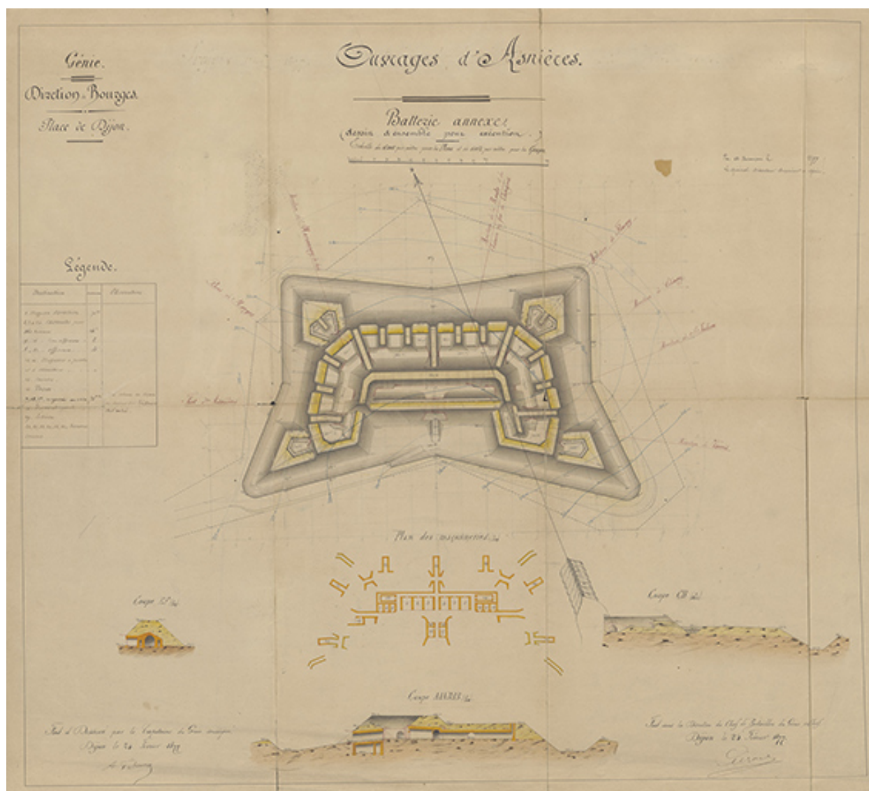
Ouvrages d'Asnières. Batterie annexe (dessin d'ensemble pour exécution). 1877.
